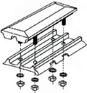
Patins à boulonner
