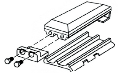
Patins à clipser
